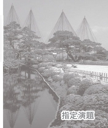
プログラム
